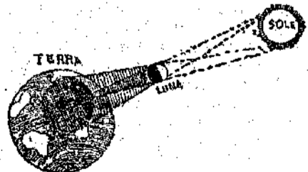
Figura teorica dell'eclisse.
