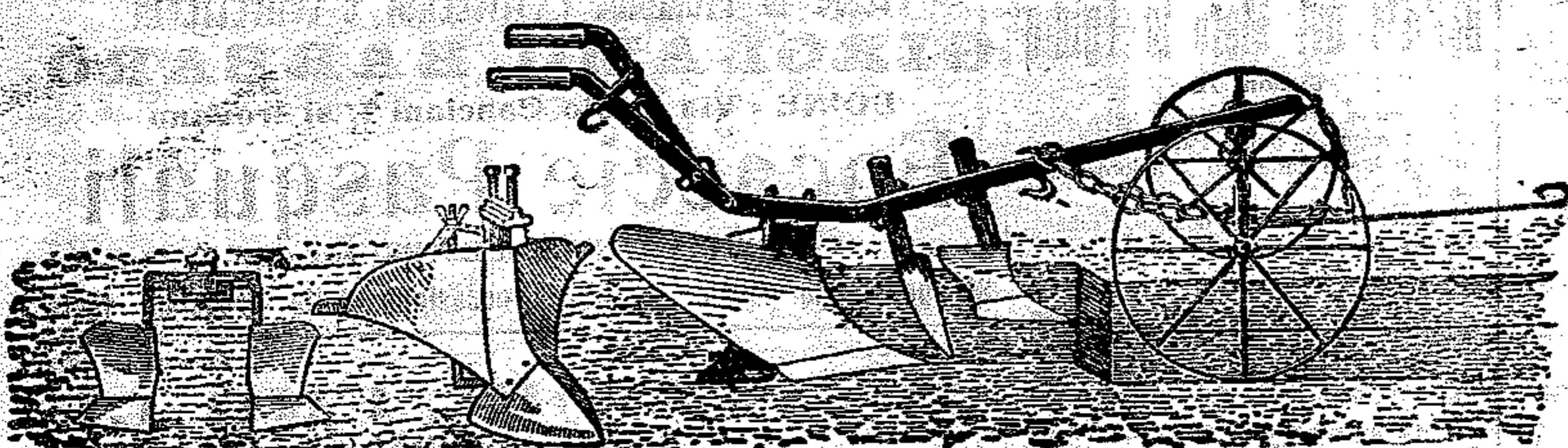
Gruppo completo su unica buca (But) per tutte le lavorazioni dei terreni (aratro completo con carrello, con rincalzatore e con zappi applicabili tutti sulla stessa buca. Prezzi per gruppi completi: N. 6 (scheletro acciaio) L. 600. - N. 7 (scheletro acciaio) L. 676. - N. 8 (scheletro acciaio) L. 750. - N. 10 (scheletro acciaio) L. 775. Centinaia di esemplari sono ininterrottamente forniti.
