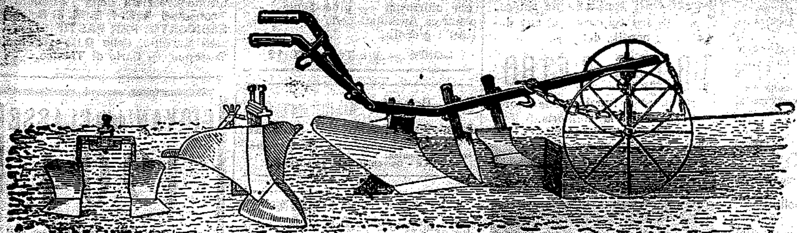
Gruppo completo su unica bure (But) per tutte le lavorazioni dei terreni aratro completo con corredo, con rincalzatore e con zappini applicabili, tutti (sulla stessa bure). - Prezzi per gruppi completi: N. 7 (scheletro) acciaio L. 675 - N. 10 (scheletro ferro forgiato) L. 725 - N. 10 scheletro acciaio L. 775 - Centinaia di esemplari sono ininterrottamente forniti.
