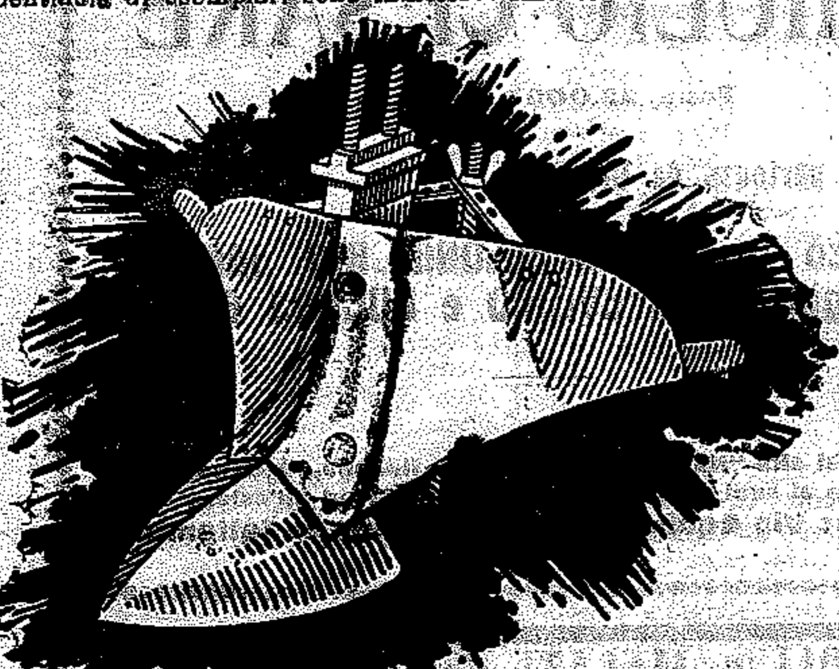
Gruppo completo su unica bure (But) pure tutte le lavorazioni dei terreni aratro completo con rincalzatore e con zappini applicabili, tutti (sulla stessa bure). - Prezzi per gruppi completi: N. 7 (scheletro) acciaio L. 675 - N. 10 (scheletro ferro forgiato) L. 725 - N. 10 scheletro acciaio L. 775 - Centinaia di esemplari sono ininterrottamente forniti.
