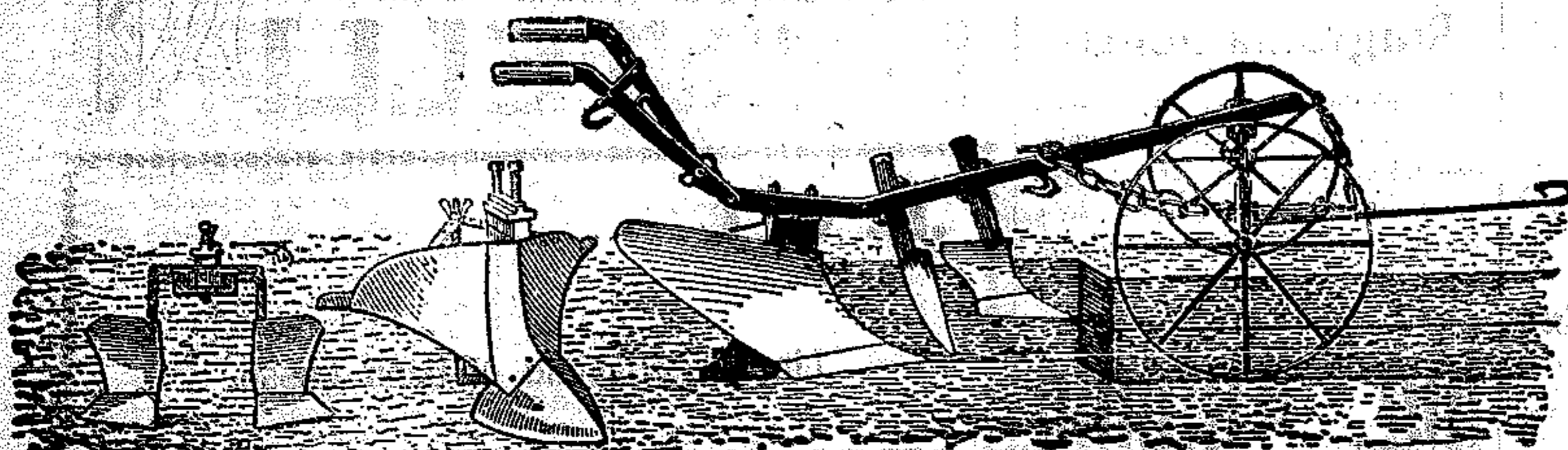
Gruppo completo su unica bure (But) pure tutte le lavorazioni dei terreni aratro completo con rincalzatore e con zappini applicabili, tutti (sulla stessa bure). - Prezzi per gruppi completi: N. 7 (scheletro) acciaio L. 675 - N. 10 (scheletro ferro forgiato) L. 725 - N. 10 scheletro acciaio L. 775 - Centinaia di esemplari sono ininterrottamente forniti.
