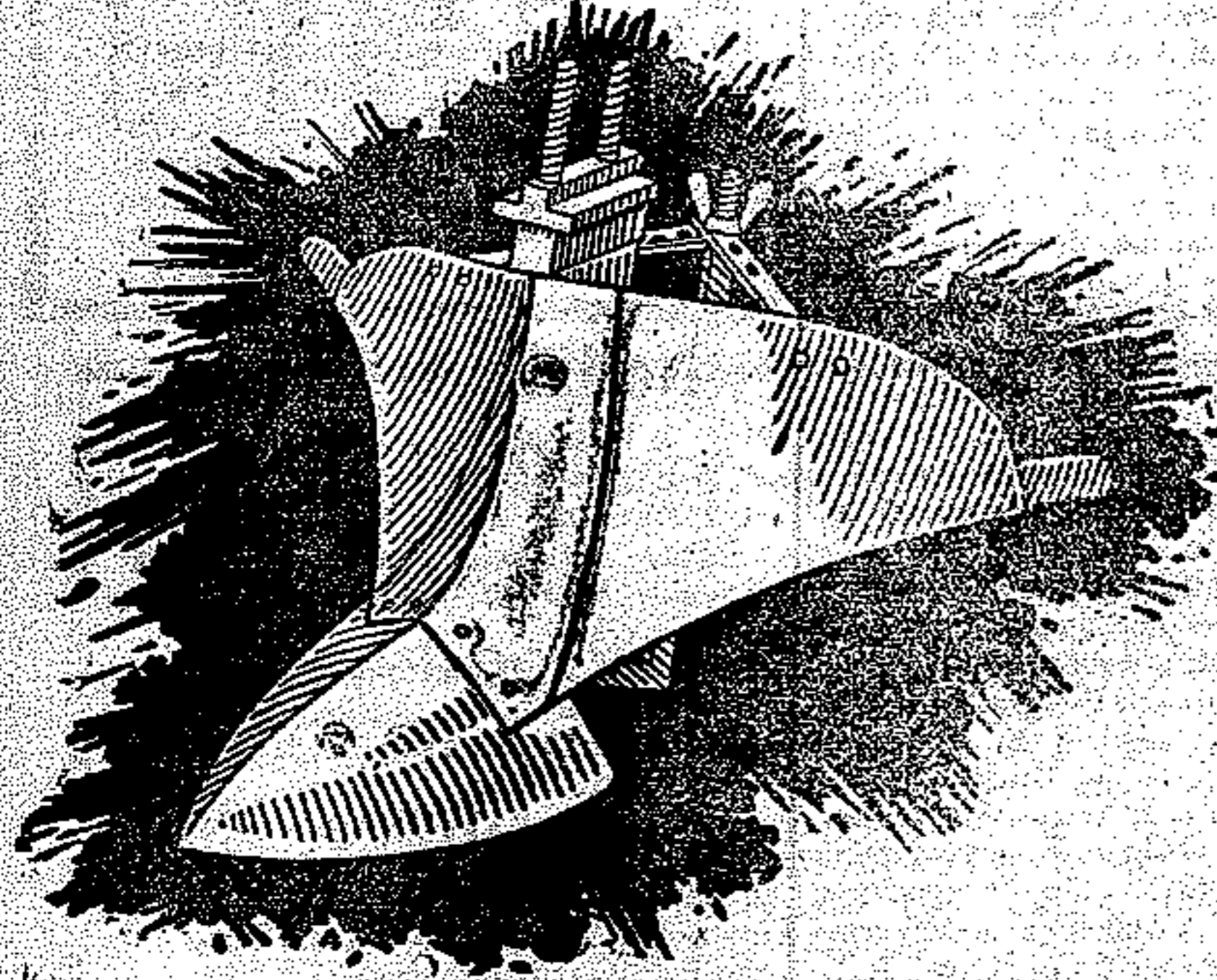
Gruppo completo su unica bure (But) per tutte le lavorazioni del terreno aratro completo con carrello, con rincalzatore e con zappini applicabili, tutti su la stessa bure) - Prezzi per gruppi completi: N. 7 (scheletro) acciaio L. 675 - N. 10 (scheletro ferro forgiato) L. 725 - N. 10 (scheletro acciaio) L. 775 - Centinaia di esemplari sono ininterrottamente foratori
