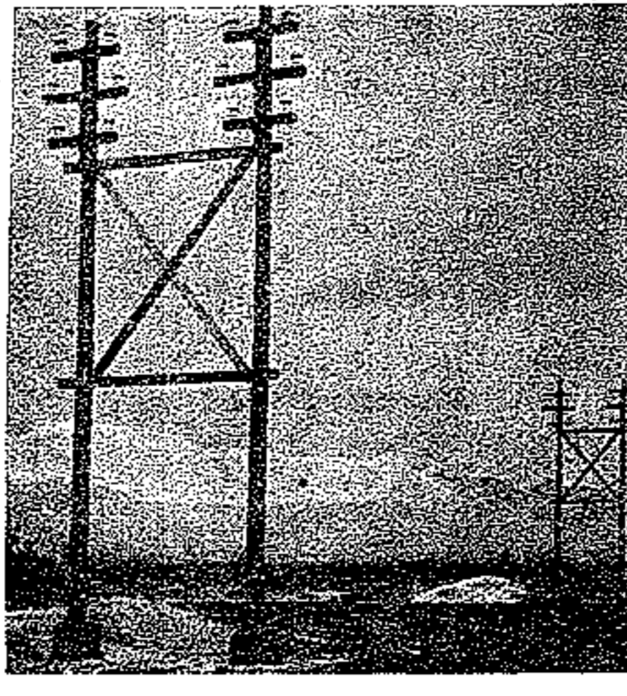
L'impianto per il trasporto della forza elettrica da Malnisio a Venezia.
