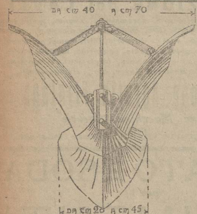
ARATRI rincalzatori applicabili a qualunque bure (bat)
