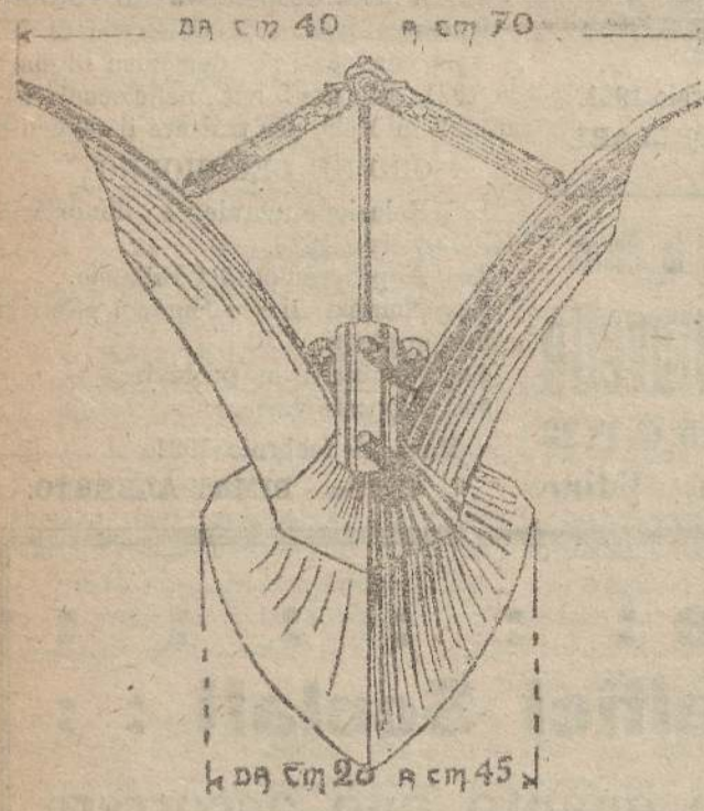
ARATRI ricalzatori applicabili a qualunque bure (bat)
