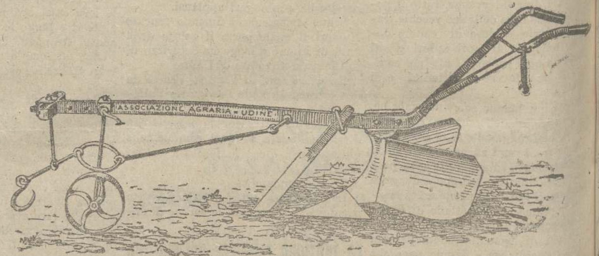
ARATRO rinalzatore
