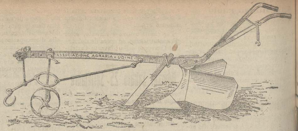
ARATRO rincalzatore
