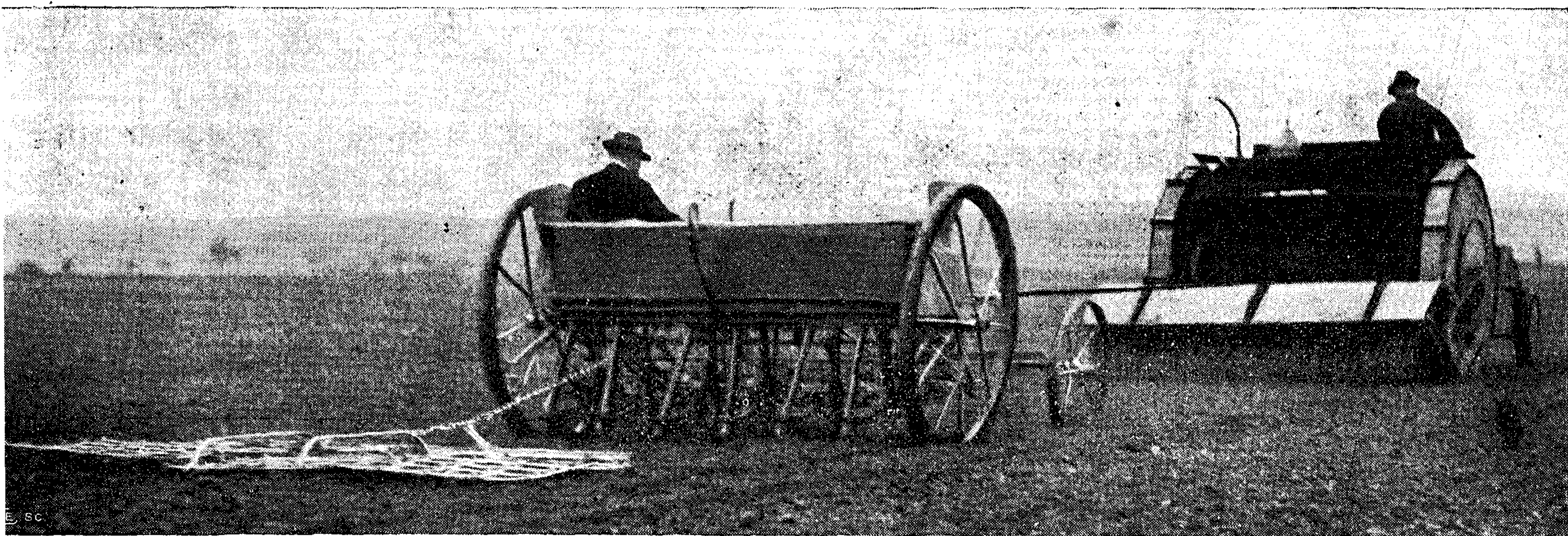
L'apparecchio di Meyenburg può compiere il lavoro di preparazione del terreno e di semina in una sol volta.
