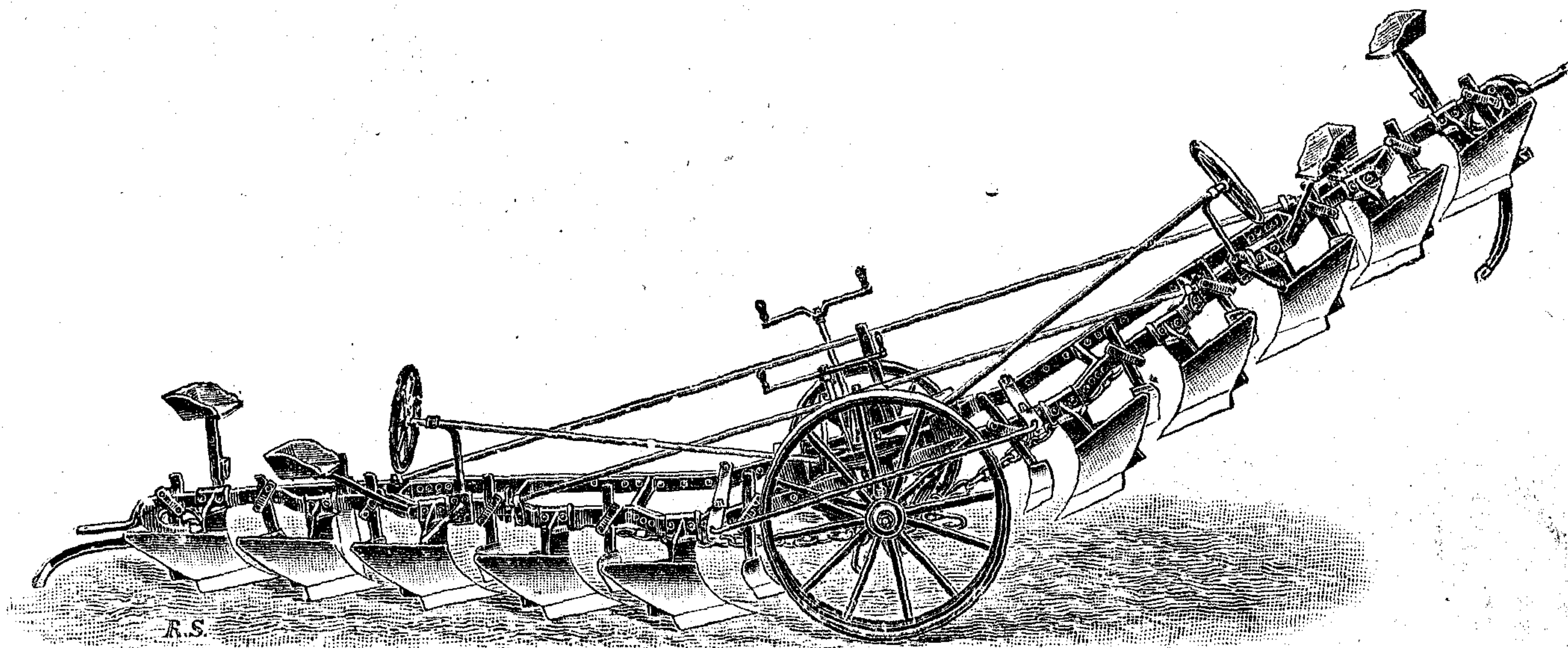
Aratro SACK a bilanciere (pentavomere).
