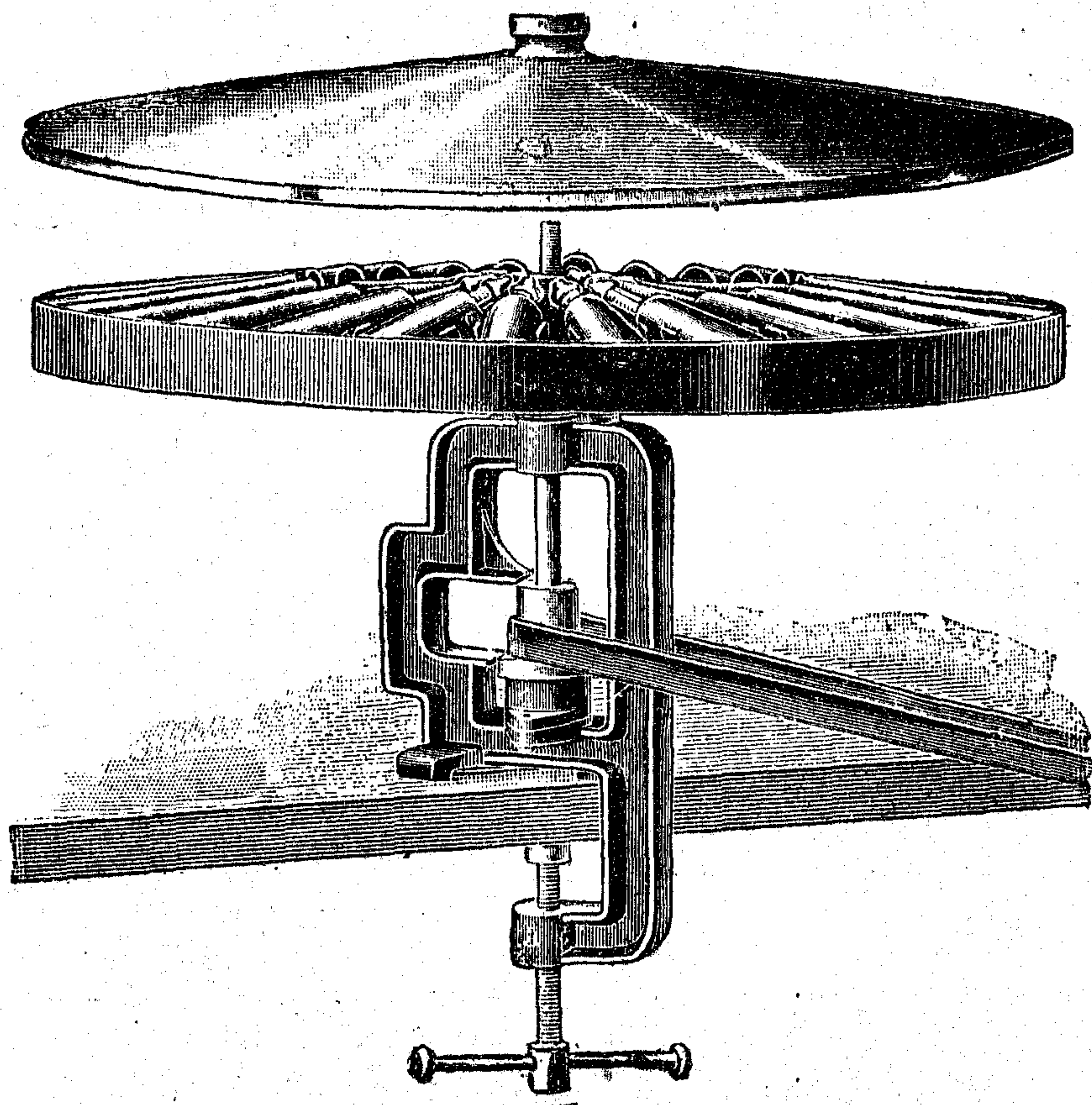
Trottola Gerber, tipo Rapid, a 16 prove per l'analisi del latte.
