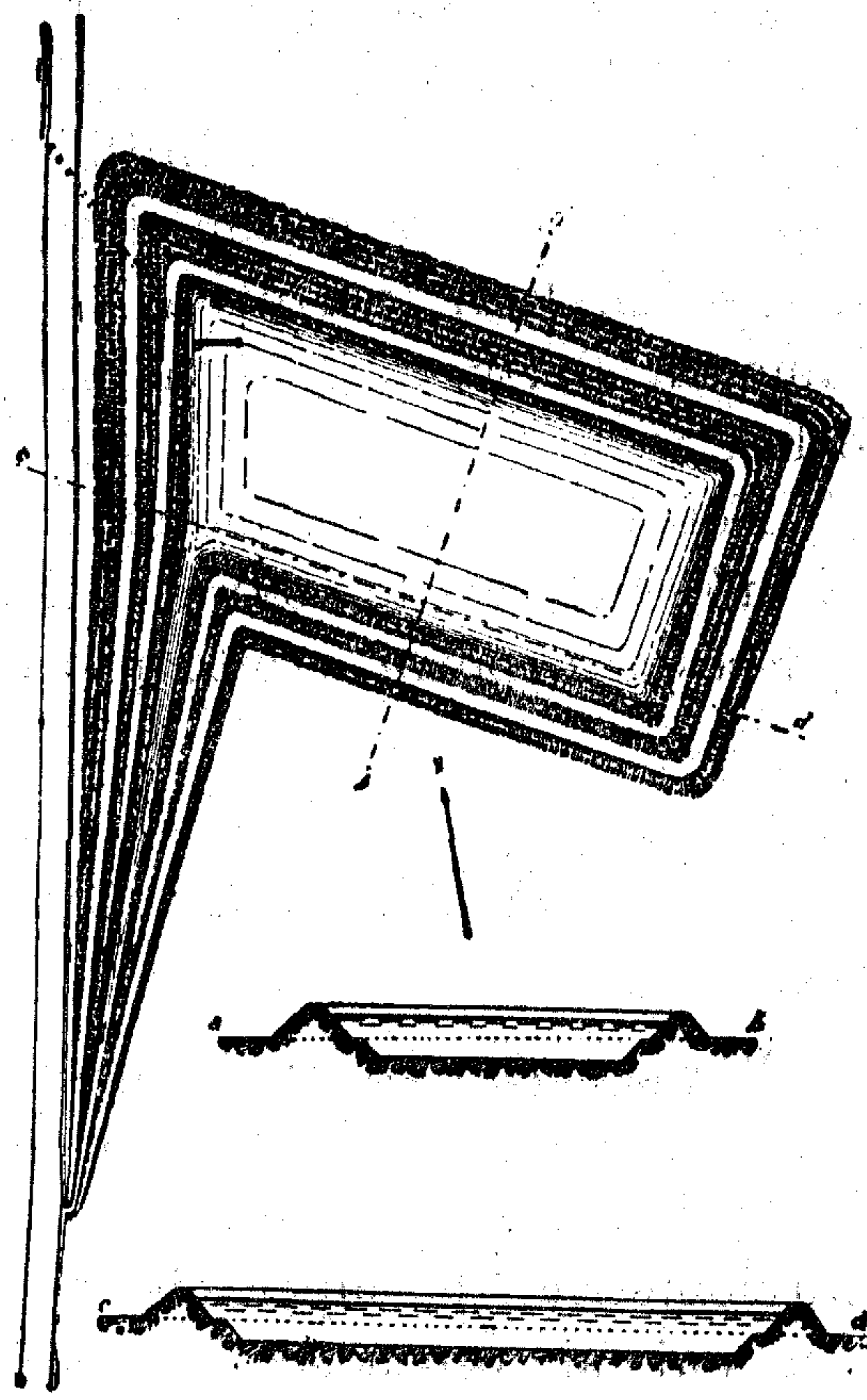
Pianta e Sezioni del Serbatoio Rivasso di Sotto.
