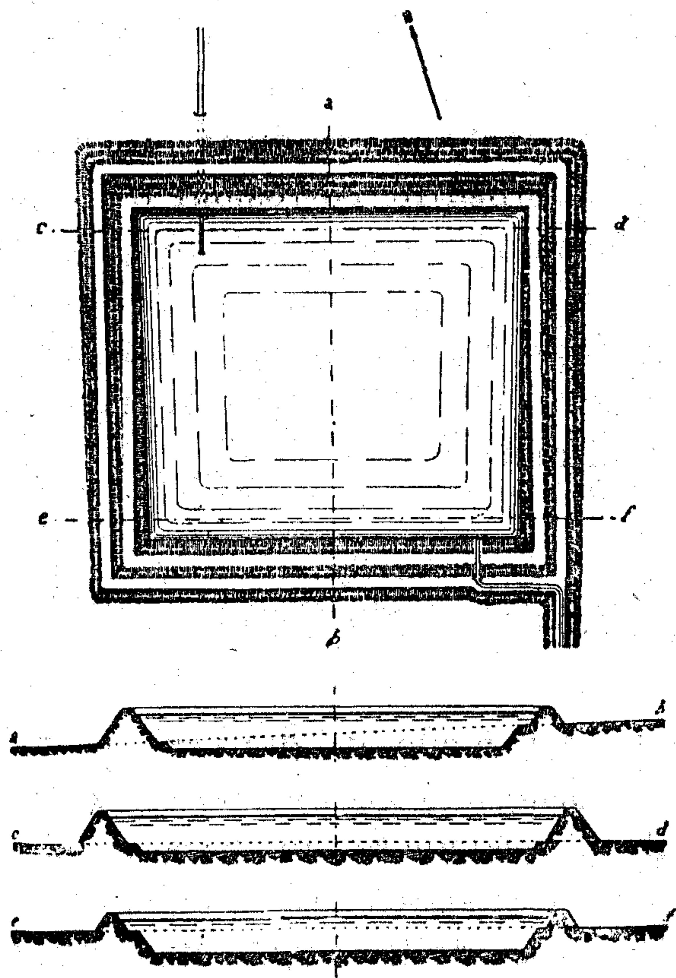
Pianta e Sezioni del Serbatoio Lische.
