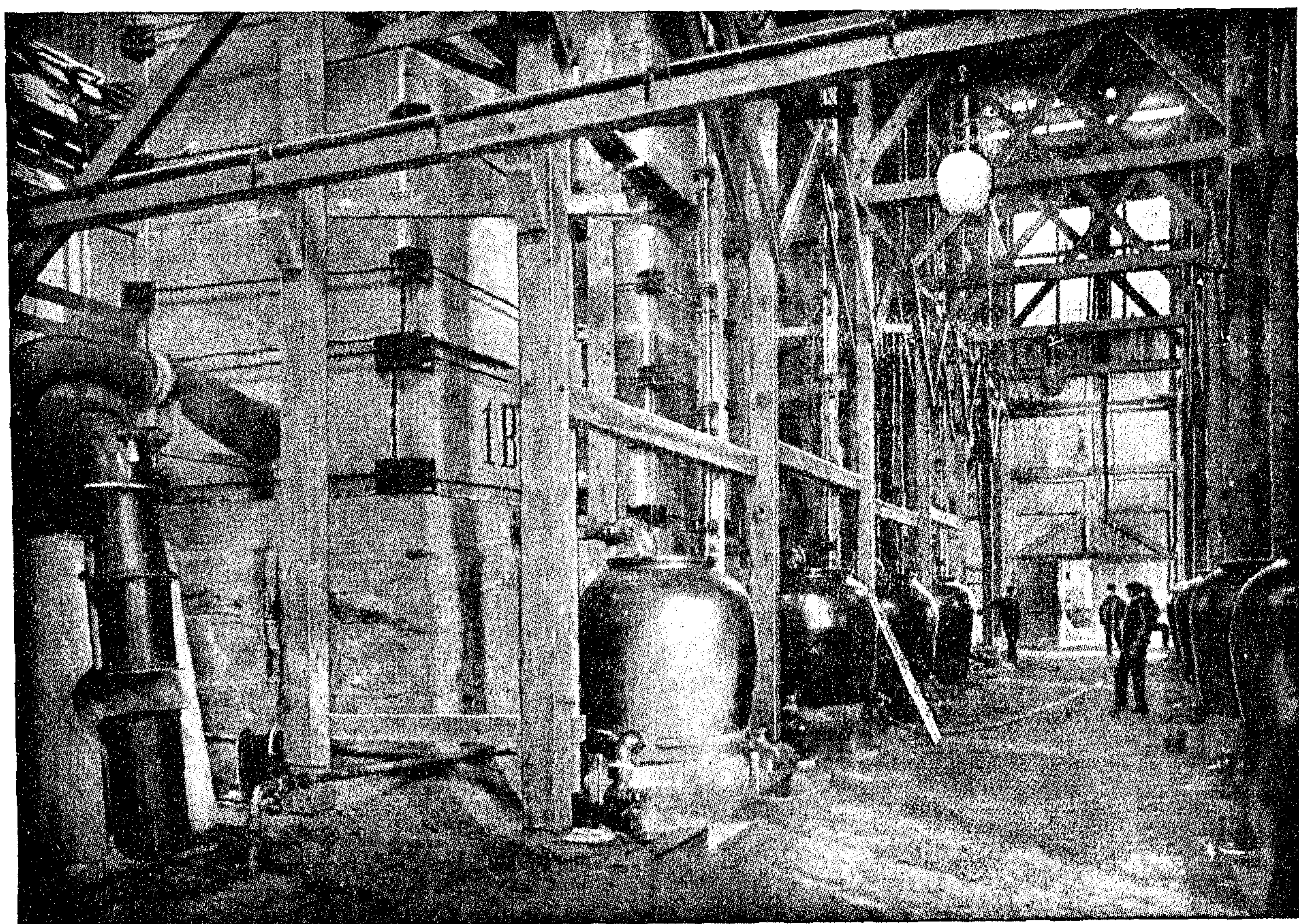
Fig. 8. a — Apparecchi d'assorbimento della fabbrica di Notodden.
