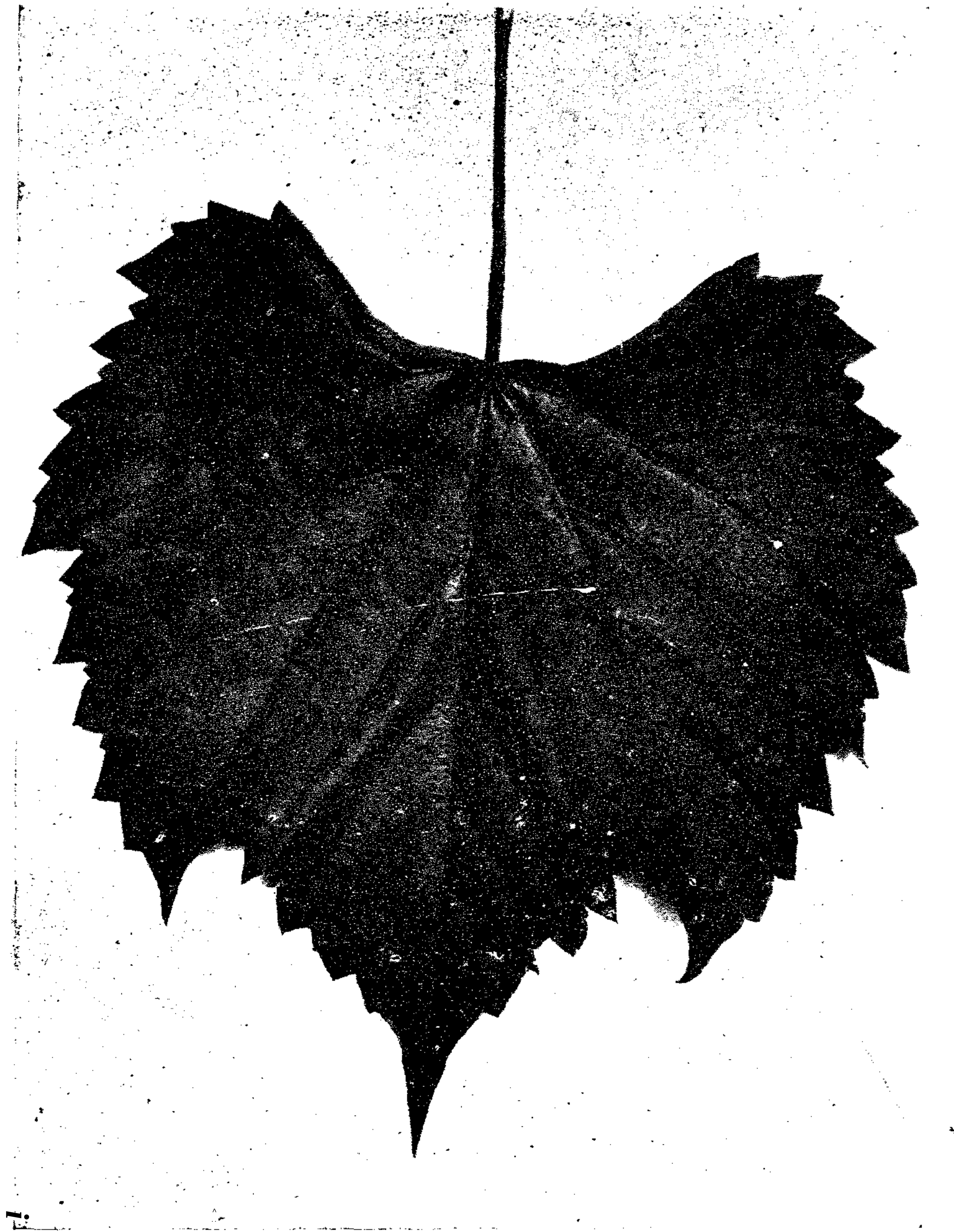
Fig. 9. — Riparia × Rupestis N. 10114 (Millardet).
