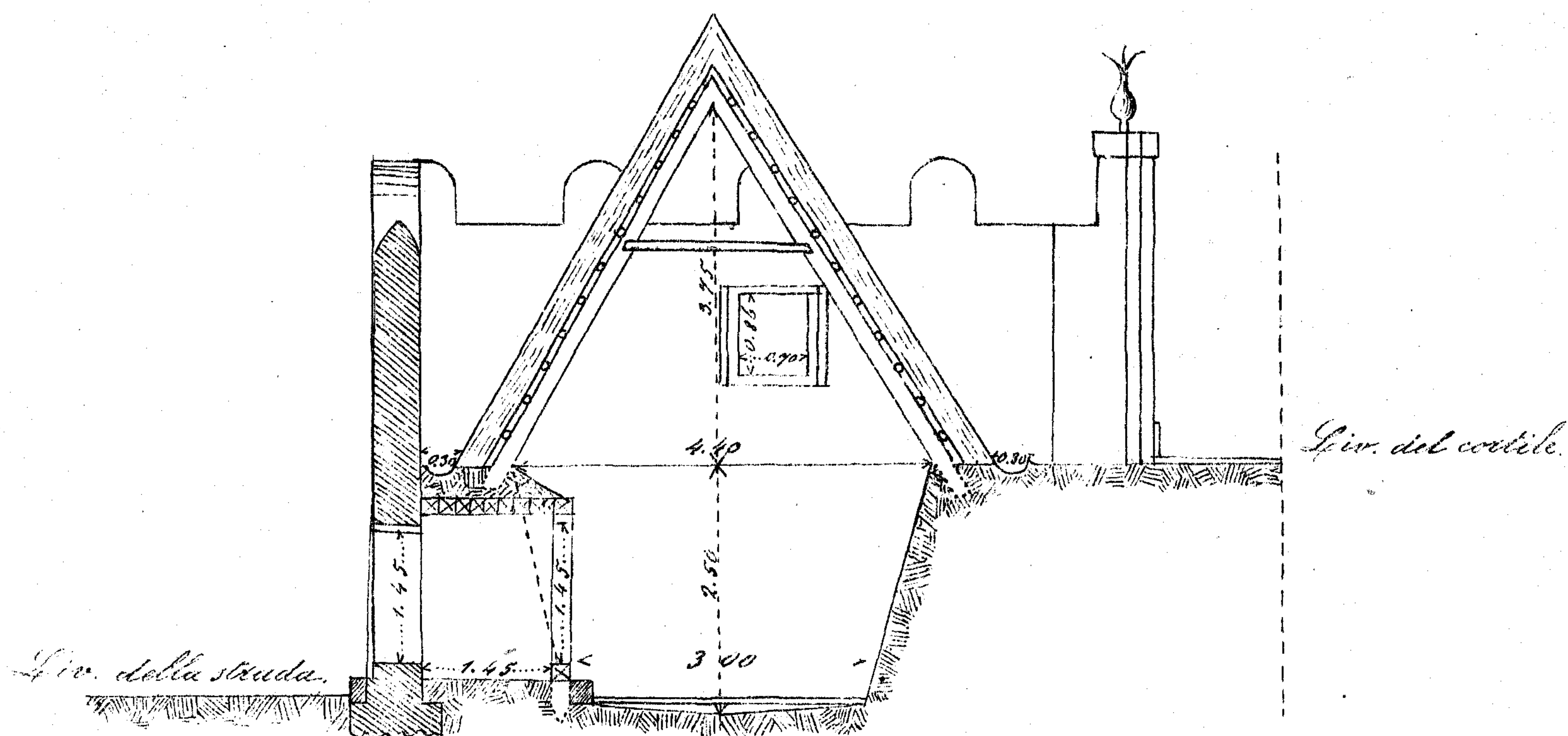
Sezione A-B
