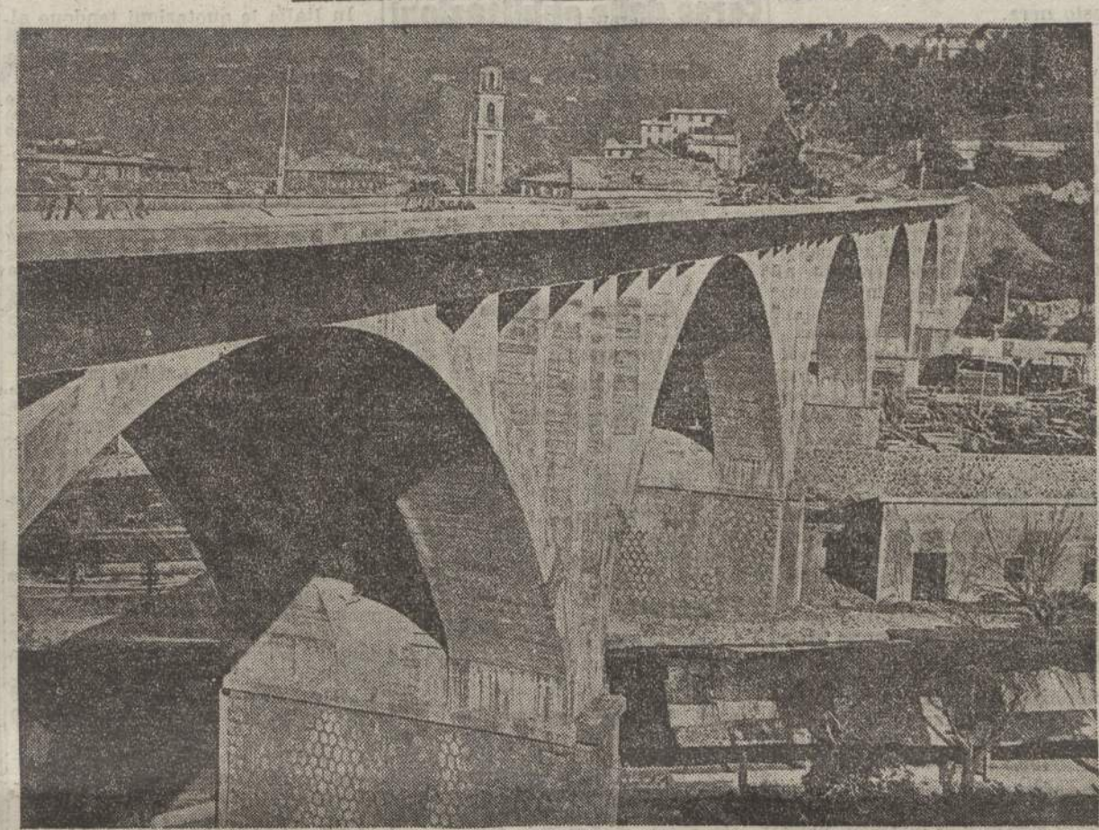
VIADOTTO TORBELLA IN 5 ARCADE DI LUCE m. 27 PRESSO RIVAROLO
