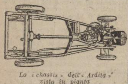
Lo « chassis » dell' « Ardita » visto in pianta
