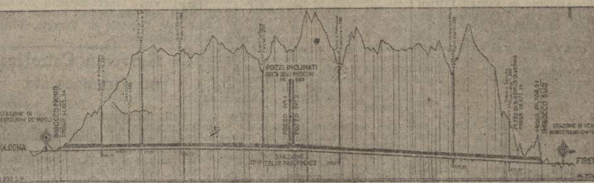
Il profilo longitudinale della Grande Galleria dell'Appennino, lunga m. 18.510. L'asterisco indica il punto ove è caduta l'ultima diaframma.
